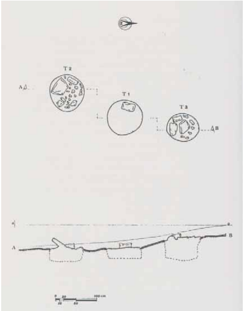
Fig 17. Planimetria e sezione delle tombe nuragiche (da Ugas)
