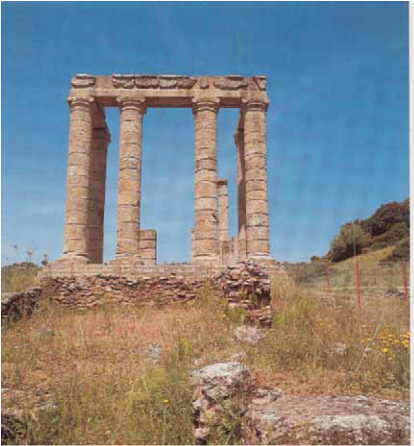
Fig 28. Antas. Ruederi dei sacelli punici incorporati nella scalinata ed il tempio del SARDUS PATER.
